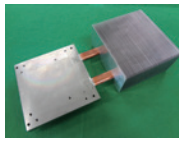
開発した新型ヒートパイプを使用したヒートシンクの例
