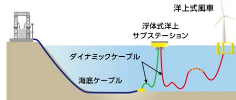
洋上式風車 浮体式洋上 サブステーション ダイナミックケーブル 海底ケーブル 浮体式洋上風力プラント用 超高压ダイナミック海底ケーブル 開発業務を受注
