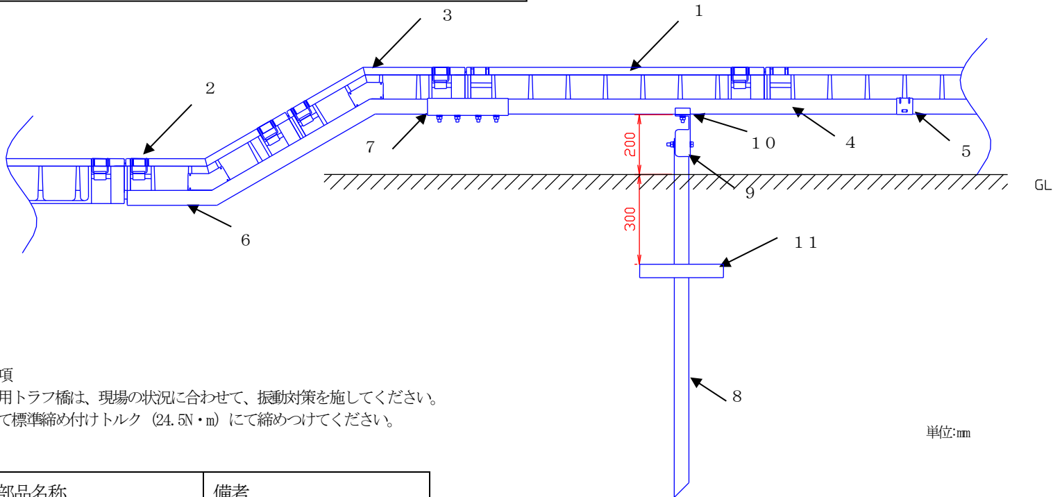
グリーントラフ用トラフ橋 立ち上がり部システム図
