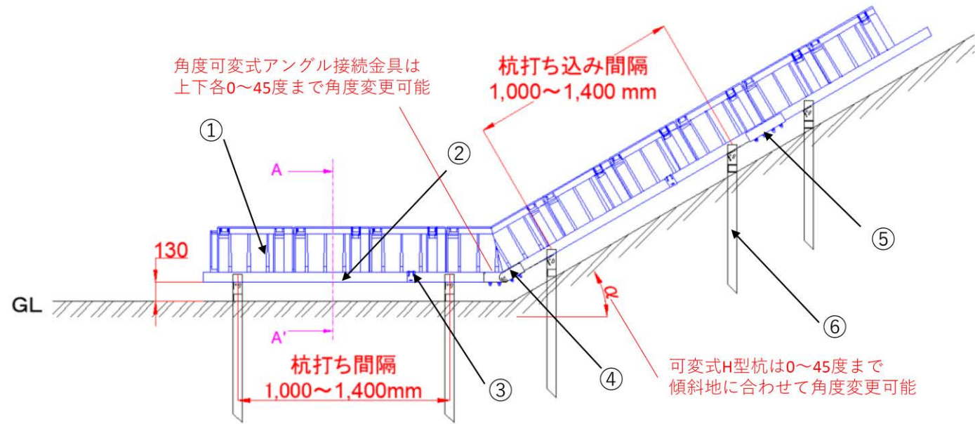
付図 9. 傾斜地対応トラフ橋 傾斜立ち上がり部 施工図例
