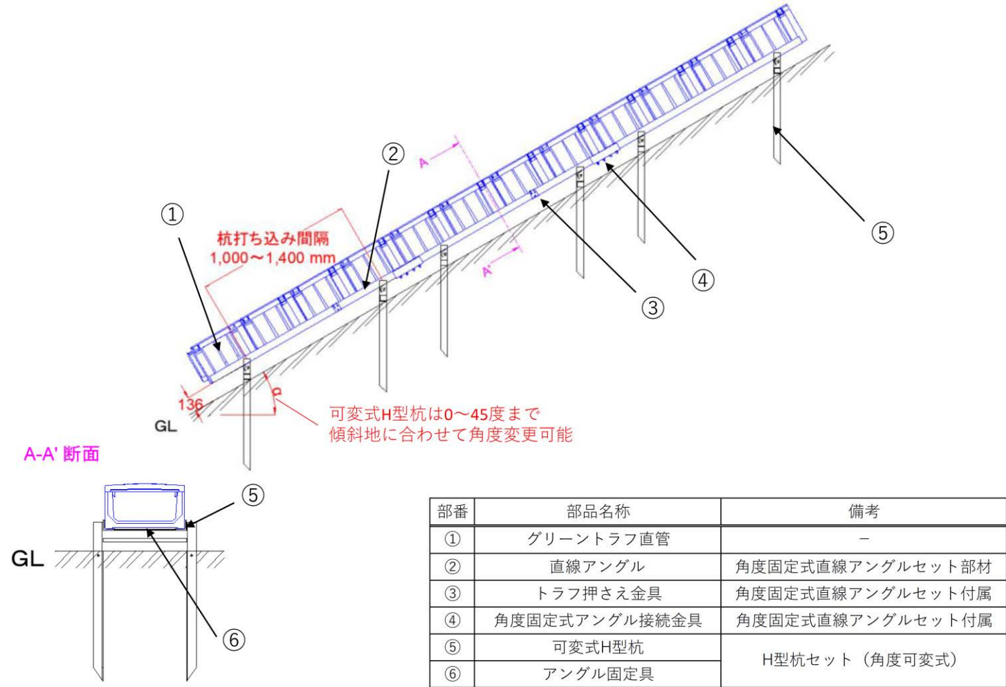
付図 11. 傾斜地対応トラフ橋 傾斜部 施工図例
