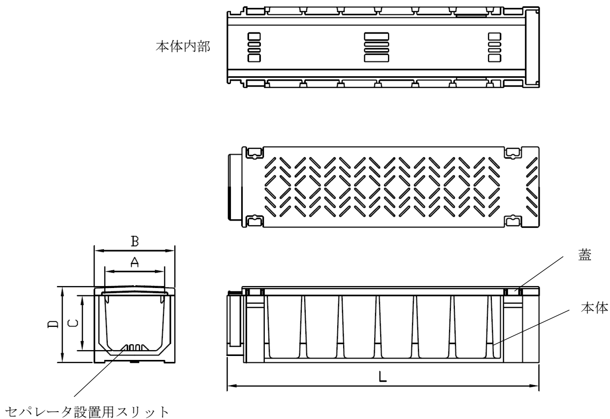
付図 2 直管 複孔式
