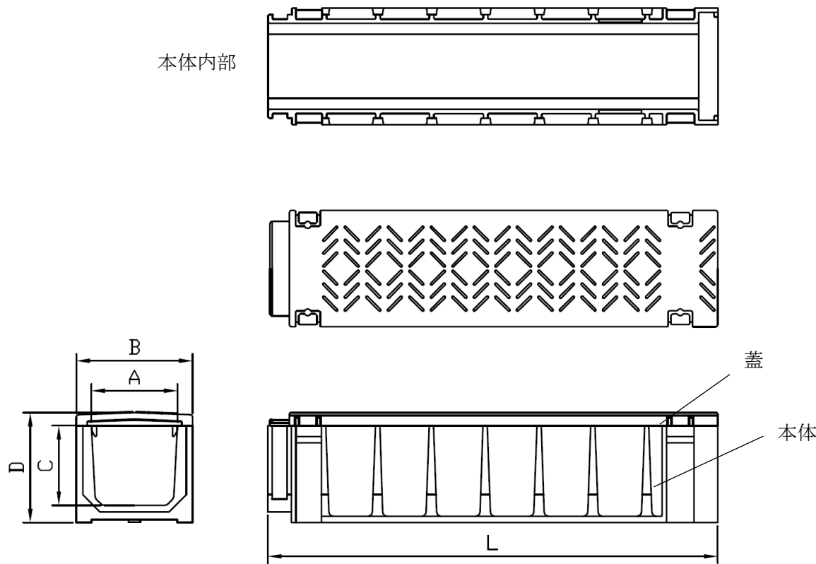
付図 1 直管
