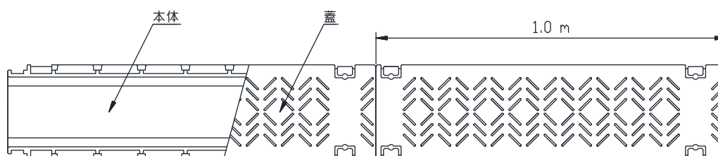
図－1 構造（120S,150B,200B,300B,300C 組図）
